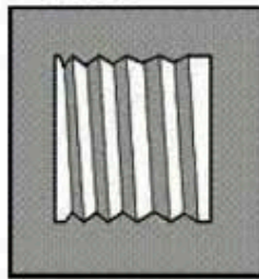
Glow plug body thread Lietatura corpo candele Rosca del cuerpo de la bujía
